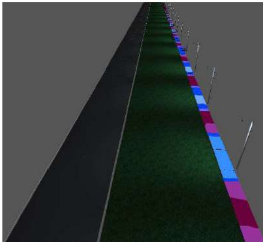
Figura 6 - Níveis de iluminância 3D da Ciclovía com Poste Solar 40W.
