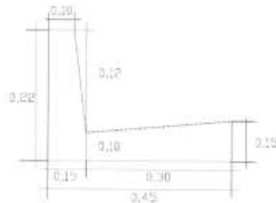
Imagem 01 – Detalhamento do perfil de guias e sarjeta extrusada - área = 0,065 m 2 .
